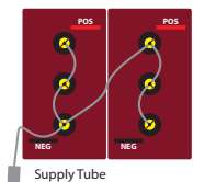
12V example with 2 - SIND 06 1225 batteries
