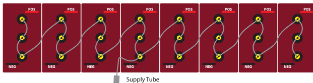
48V example with 8 - SIND 06 1225 batteries
