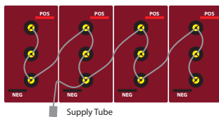
24V example with 4 - SIND 06 1225 batteries
